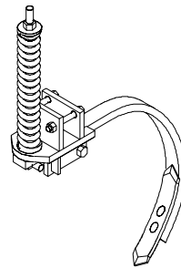
CP chisel tyne
